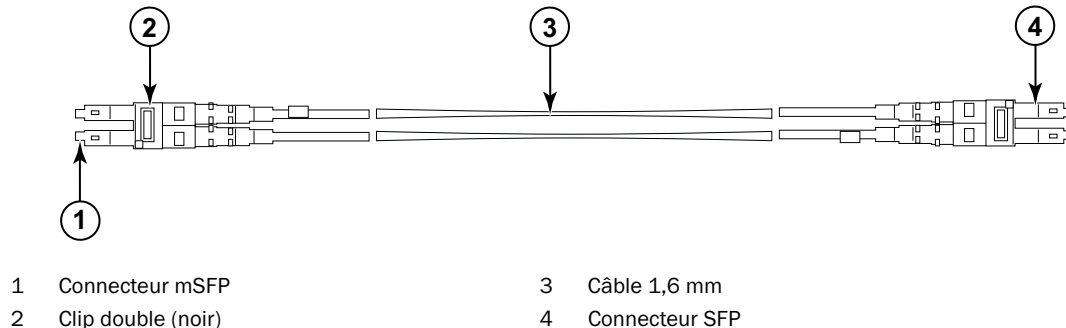
FIGURE 6 Conception de câble pour les câbles de raccordement mSFP pour la lame FC8-64 à port haute densité
